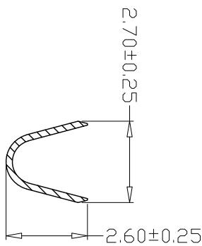
SEC: A-A
